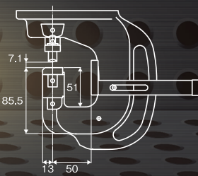
寸法図
