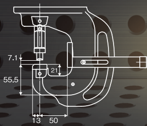
寸法図
